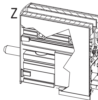
Stirnfeststeller Locating pin Erdot de verrouillage
