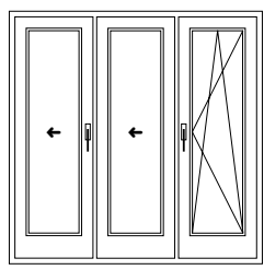
Schema 321 [1] 2 ante scorrevoli a libro, 1 anta-ribalta
