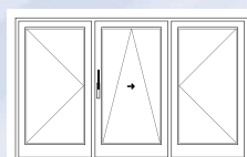
Schema G – con montante [1] 1 porta scorrevole in parallelo a ribalta, 2 porte con apertura a bandiera disegno: montaggio sinistro
