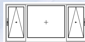
Schema K – con montante 2 scorrevoli in parallelo a ribalta, 1 vetro fisso; disegno: montaggio sinistro e montaggio destro
