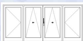
Schema C – con montante [1] 2 porte scorrevoli in parallelo a ribalta, 2 porte con apertura a bandiera; disegno: battente principale con montaggio sinistro
