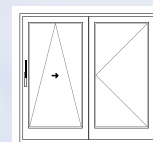
Schema D – senza montante [2] 1 porta scorrevole in parallelo a ribalta, 1 porta con apertura a bandiera; disegno: montaggio sinistro
