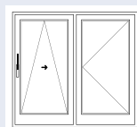
Schema A – con montante [1] 1 porta scorrevole in parallelo a ribalta, 1 porta con apertura a bandiera disegno: montaggio sinistro
