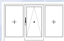
Schema G – con montante 1 scorrevole in parallelo a ribalta, 2 vetri fissi; disegno: montaggio sinistro
