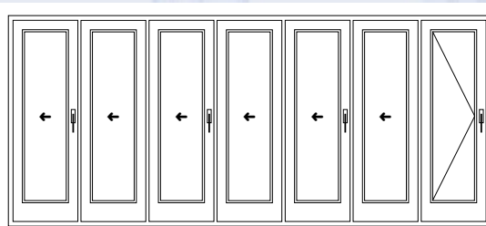
Schema 770 6 ante scorrevoli a libro, 1 anta con apertura a bandiera
