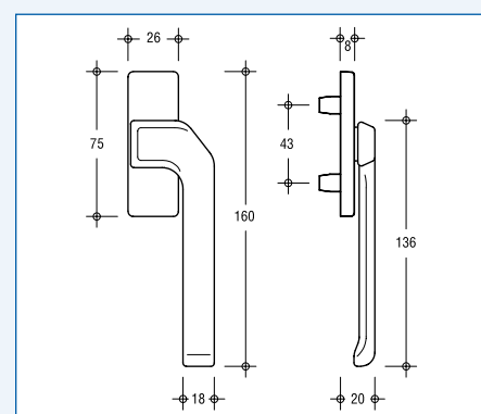
DIRIGENT-F/AGF (dargestellt: DIN links)
