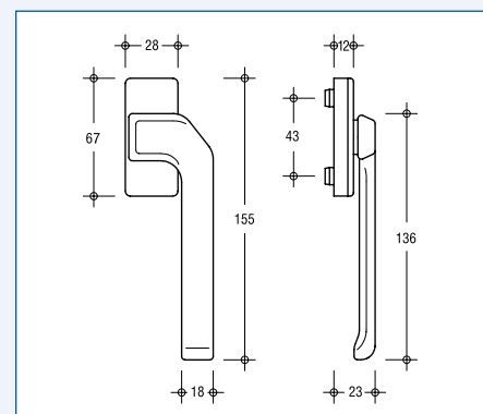
DIRIGENT-F/GF (dargestellt: DIN links)
