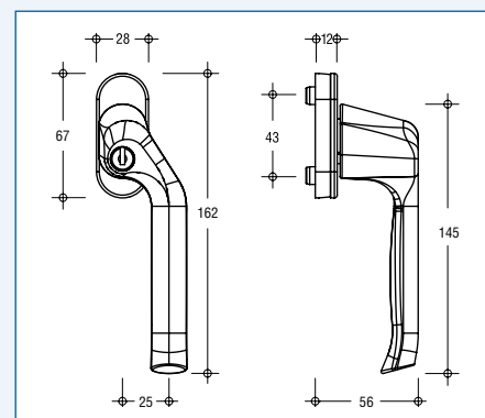
ADAGIO-F/GZ (dargestellt: DIN links)
