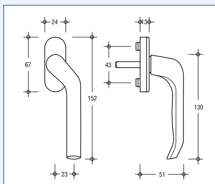
ADAGIO-F/G 24 (dargestellt: DIN links)
