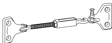
Aggancio per doppio serramento ATLAS-B
