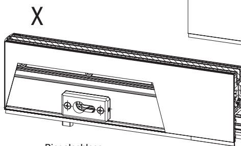
Riegelschloss Deadlock Serrure à pêne dormant
