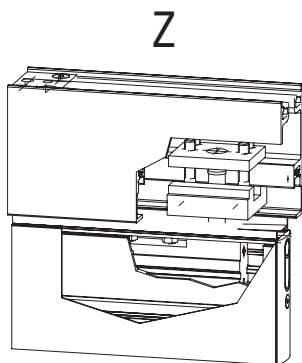
Oberer Drehpunkt Top pivot point Axe de rotation haut
