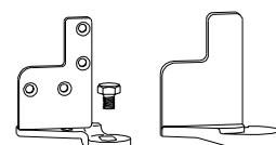
Supporto angolare 6-25337-00-L-3
