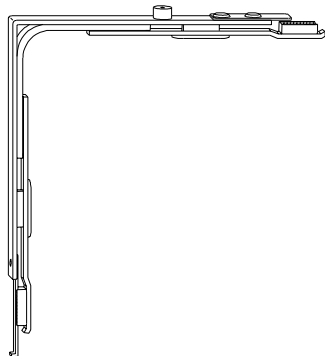
Trasmissione angolare superiore 6-25461-01-0-3
