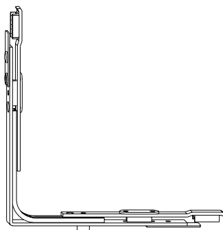
Trasmissione angolare 8-00874-00-0-3
