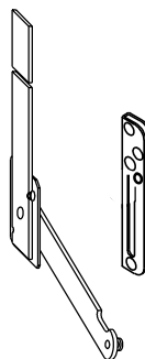
Limitatore con chiave esagonale 5-21306-00-L/R-3
